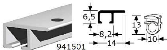
voor aluminium gordijn-rails, zie blad F-930
