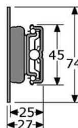
voor roestvrijstalen ondergeleidingen op kogels lopend, zie blad Y-926
