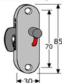
voor roestvrijstalen bezet- sluitingen voor schuifdeuren, zie blad Y-519
