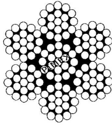
staaldraadkabel RVS, Y-160 (groep 1)
